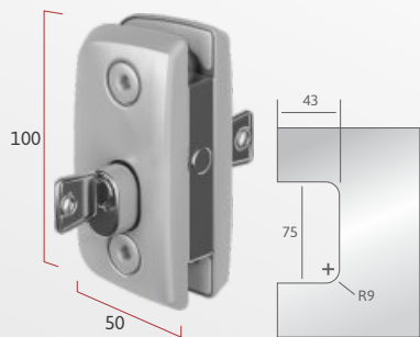
IP 1520 | 1 unidade Fechadura para porta de abrir
