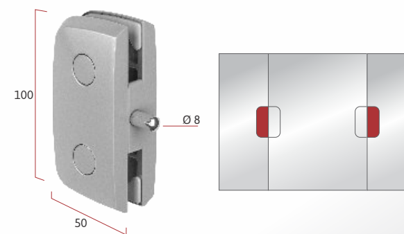
IP 1130 Dobradiça para basculante grande
