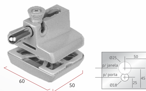
IP 1335 | 1 unidade Trinco sem miolo
