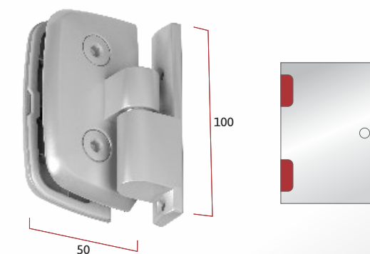
IP 1114 Dobradiça automática para box V/A
