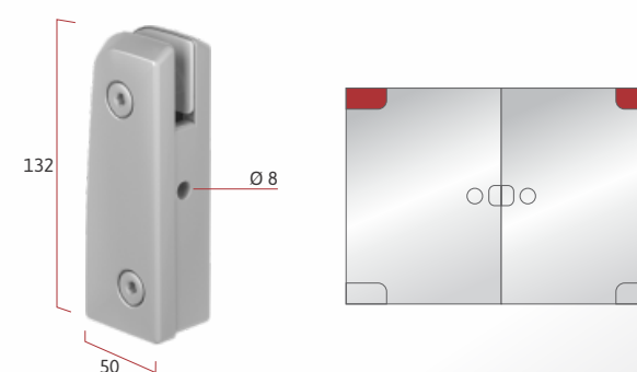
IP 1101A Dobradiça inferior com regulagem para pivô invertido
