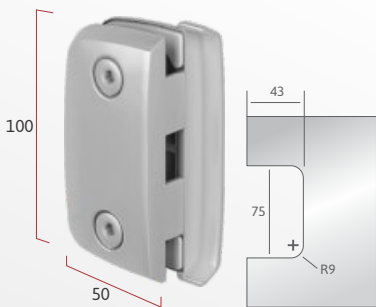
IP 1531 | 1 unidade Contra fechadura com aparador para 1520
