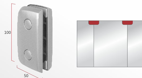
IP 1304 Suporte sem miolo para união de 02 vidros
