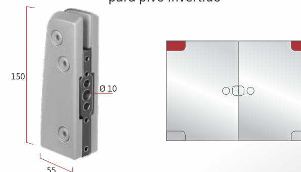
IP 1103A Dobradiça inferior com regulagem para pivô invertido
