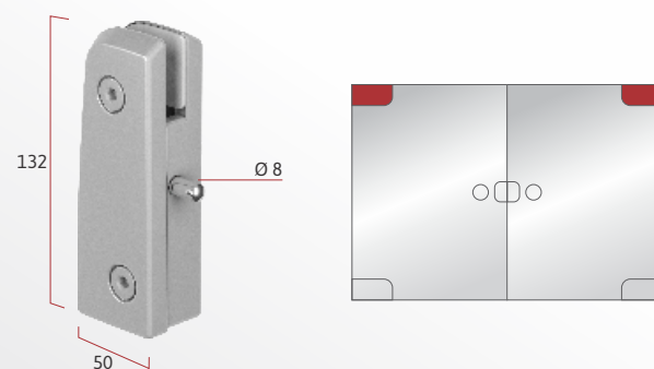
IP 1101 Dobradiça superior
