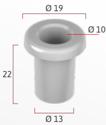
IP 1038 | 1 unidade Capuchinho para trinco com furo 10mm
