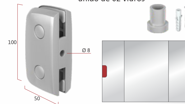
IP 1306 Suporte com miolo para união de 02 vidros
