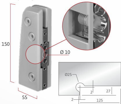
IP 1103A | 2 unidades Dobradiça inferior com regulagem para pivô invertido
