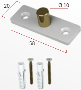
IP 1013A | 2 unidades Pivô para dobradiça com pino fixo
