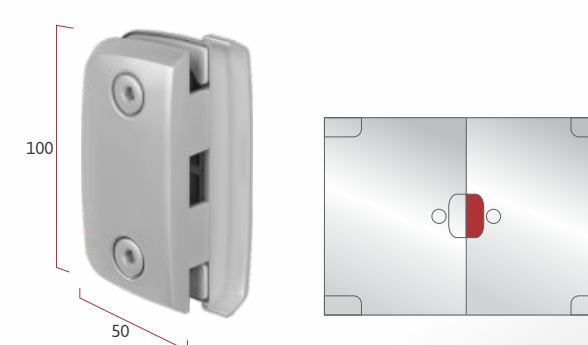
IP 1531 Contra fechadura com aparador para 1520
