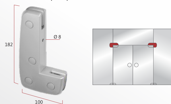
IP 1209 Facão Simples para Lateral e Bandeira
