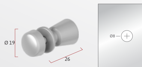
IP 1629JA | 1 unidade Puxador com 19mm de diâmetro
