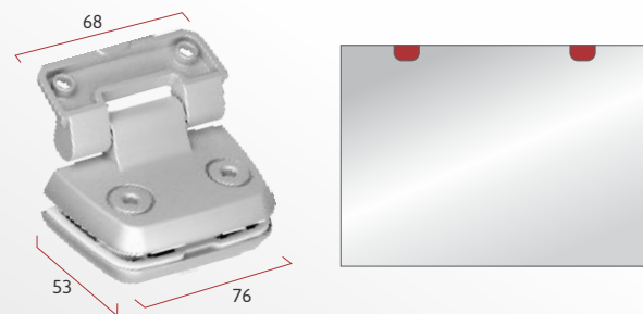
IP 1203 Suporte para bandeira com ponto de giro para dobradiça superior
