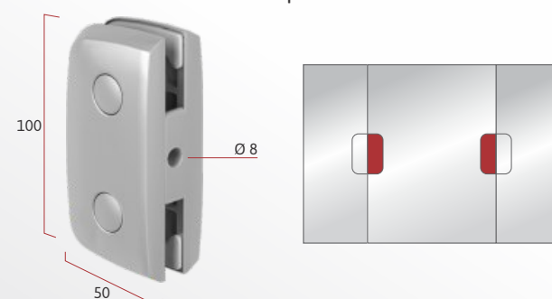
IP 1231 Suporte com ponto de giro para basculante e pivotante
