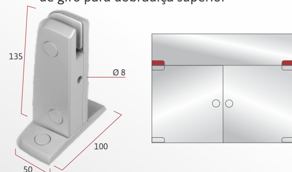
IP 1203 Suporte para bandeira com ponto de giro para dobradiça superior
