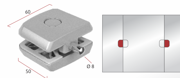
IP 1123 Dobradiça para vidro basculante
