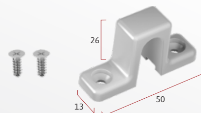
IP 1038C | 1 unidade Capuchinho para trinco (ferradura)
