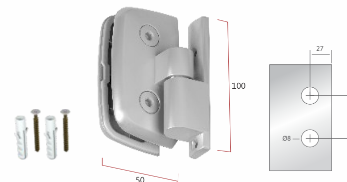
IP 1114 | 02 unidades Dobradiça automática para box V/A
