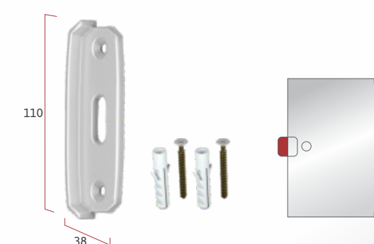
IP 1504A Contra fechadura alvenaria
