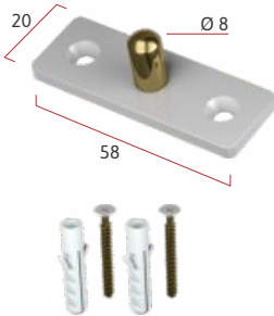
IP 1201A | 2 unidades Bucha para pivô de dobradiça
