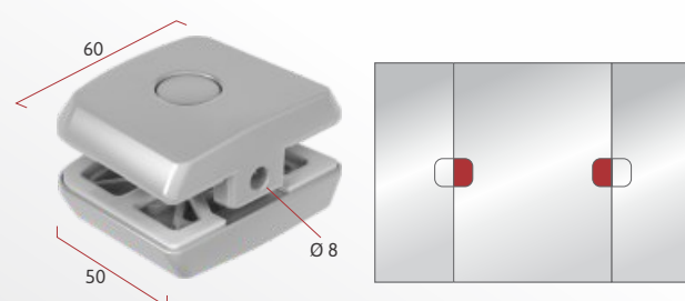
IP 1230 Suporte para basculante
