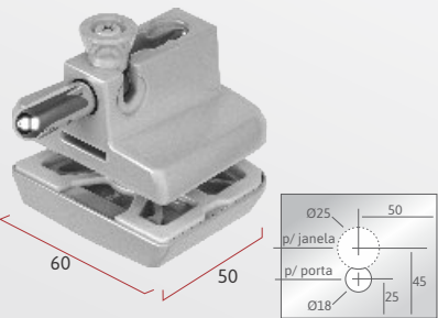
IP 1335 | 1 unidade Trinco sem miolo
