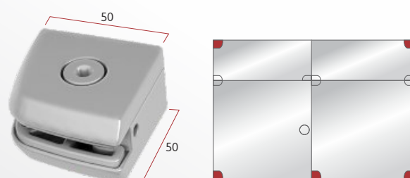
IP 1302 Suporte de Canto
