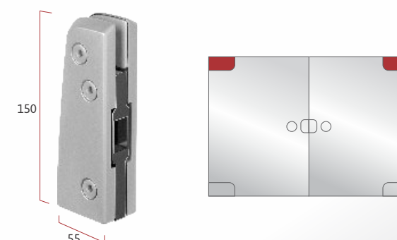
IP 1103 Dobradiça inferior para mola hidráulica
