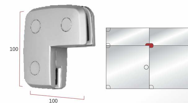
IP 1310 Suporte para união de 02 ou 03 vidros em L
