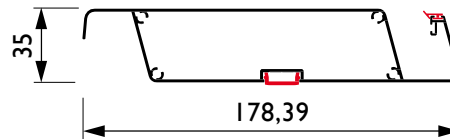
Lâmina P-150 LED ■ 050210
