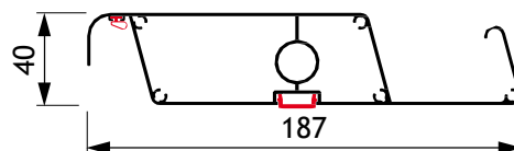
Lâmina P-190 LED ■ 050189
