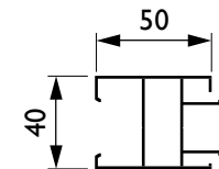
Adaptador de encaixe 40x50 mm SOFT 050218
