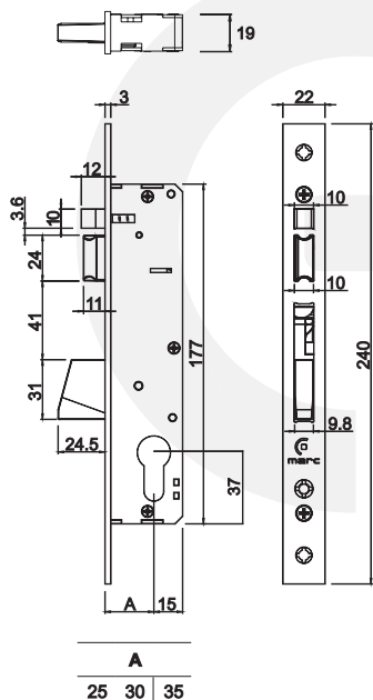
MR 733 FECHADURA ELÉTRICA
