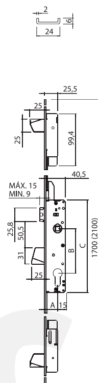
MR 750U.30 FECHADURA DE GIRO CANIVETE TRIPLA COM CONTRA TESTA 24MM
